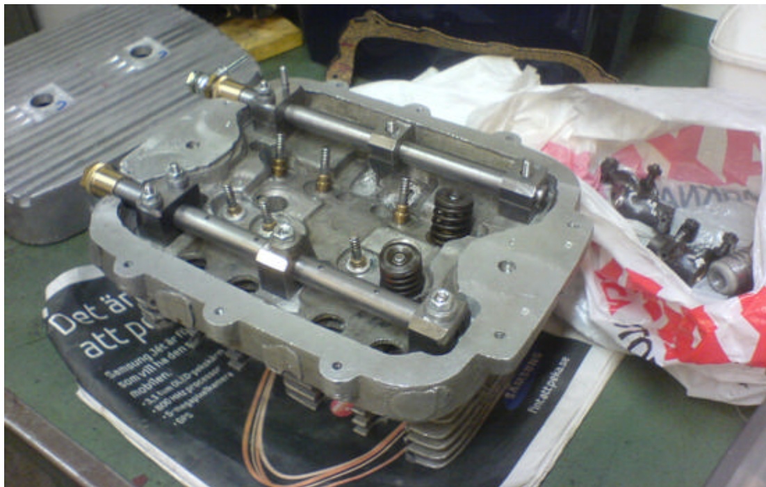
Topplöck ursprungligen från VW 1600, nu med 4 ventiler per cylinder.
